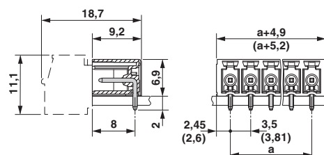
外形寸法
