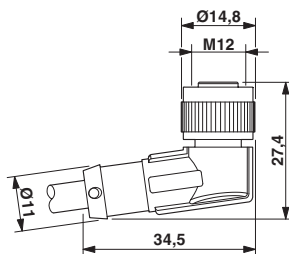
外形寸法
