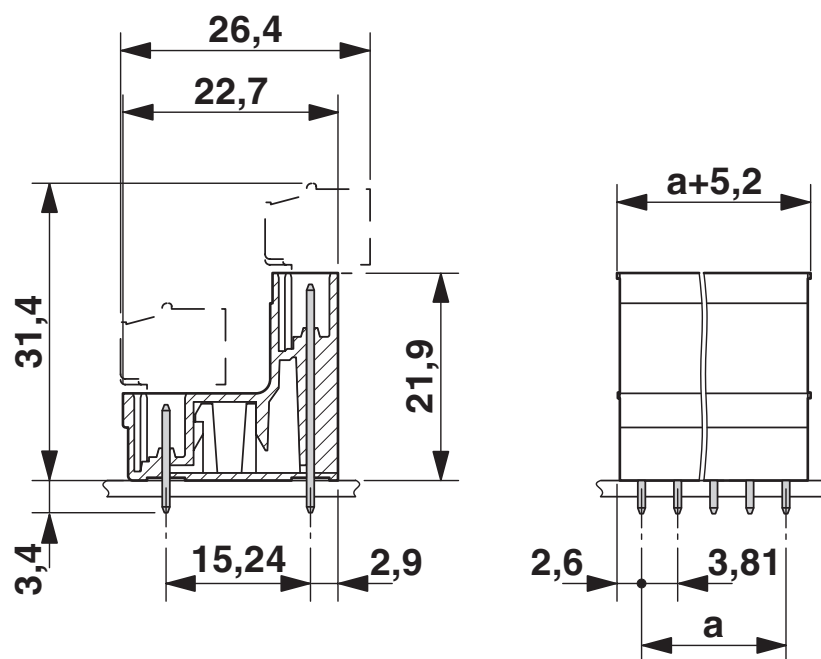
尺寸图
