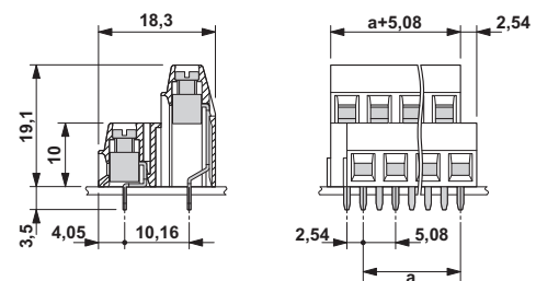
外形寸法
