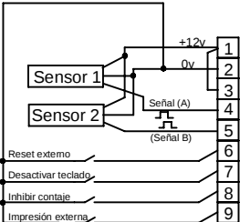
Uso ilustrado de dos sensores para proporci las señales A y B (modo de carga)
