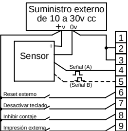
Uso ilustrado del suministro eléctrico extern (modo de generador).
