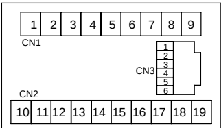
Hintere Ansicht der Klemmanordnung
