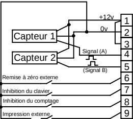
Deux capteurs A et B (mode NPN)
