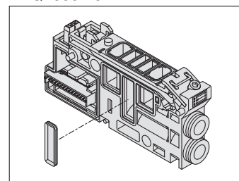
Piastra di blocco alimentazione VVQ2000-16A
