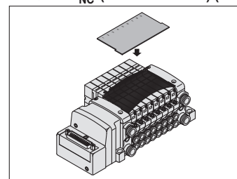
Targhetta identificativa [-N] VVQ1000-N C (-1 a max. stazioni) (-X4)
