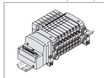
Supporto per guida DIN[-D]VVQ1000-57A {Per i kit F/L/M/P/S (EX500)} VVQC1000-57A-S {Per il kit S (EX250)} VVQC1000-57A-T (Per il kit T)
