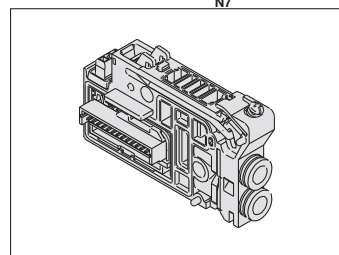
Piastra di blocco scarico VVQC1000-19A-S C3, C4 D C6, M5 N N1, N3 N 7
