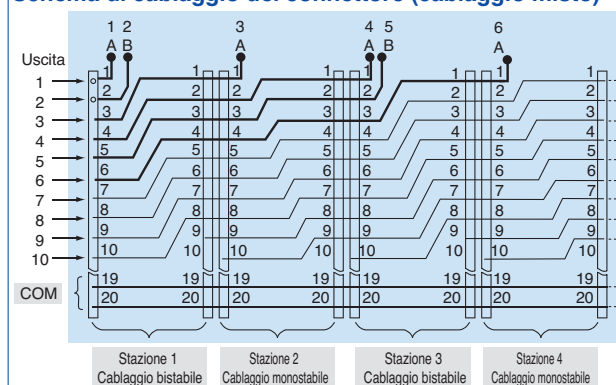
Schema di cablaggio del connettore (cablaggio misto)
