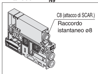
Bloccetto di scarico individuale VVQ2000-R-1-C 8 N 9
