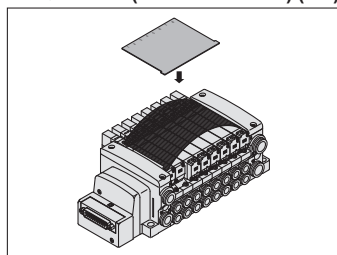
Targhetta identificativa [-N] VVQ2000-N-(1 a max. stazioni) (-X4)
