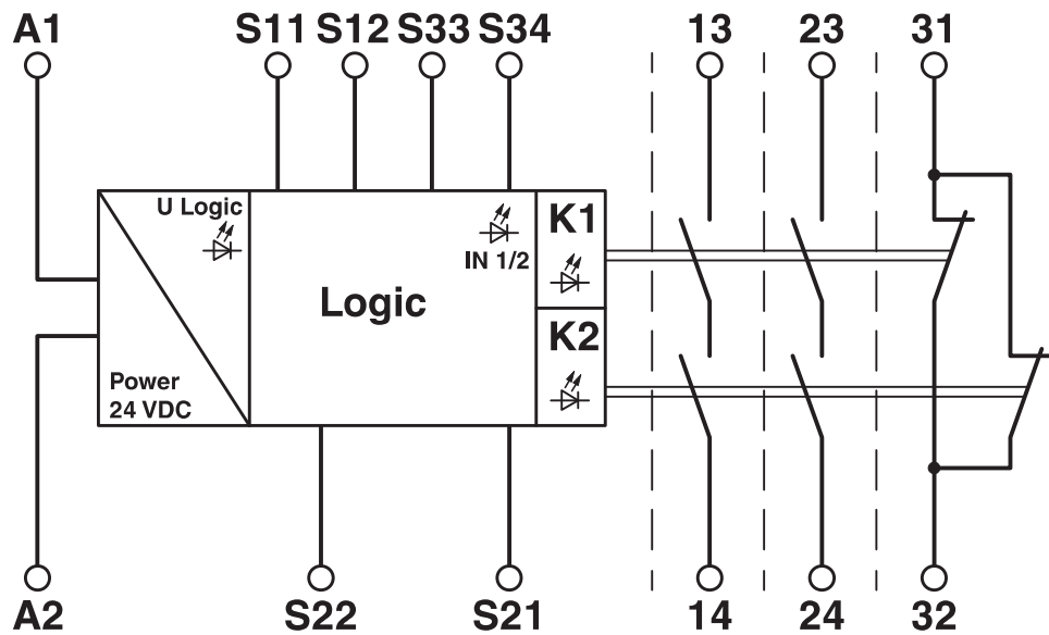
电路图
