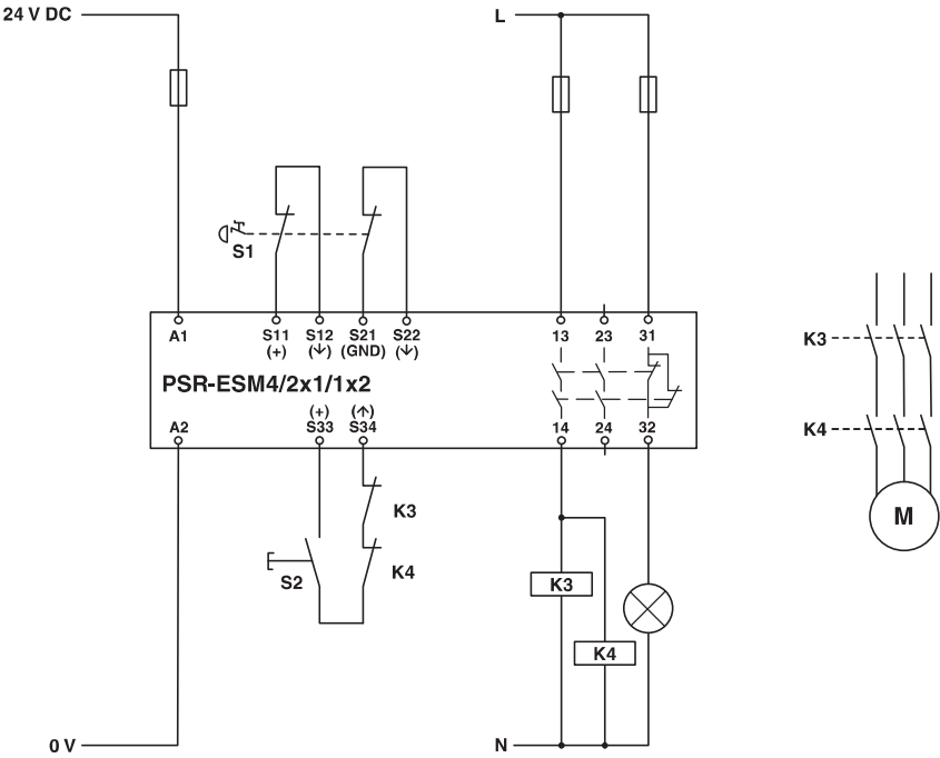
电路图
