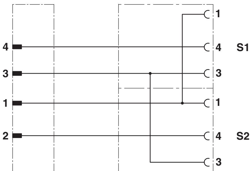
电路图
