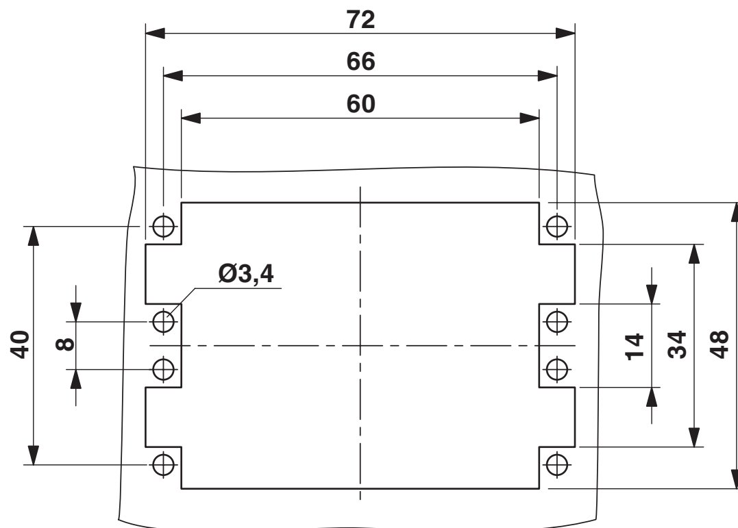
尺寸图
