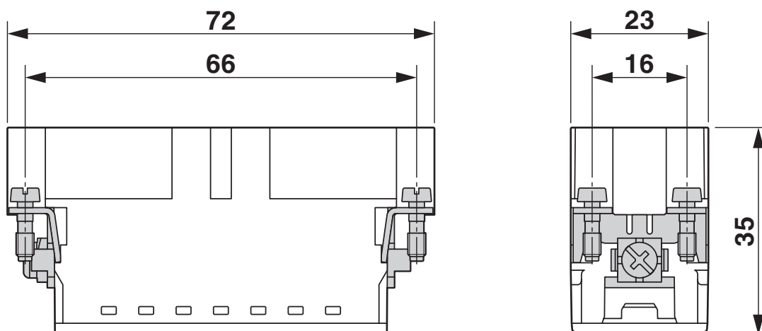
尺寸图
