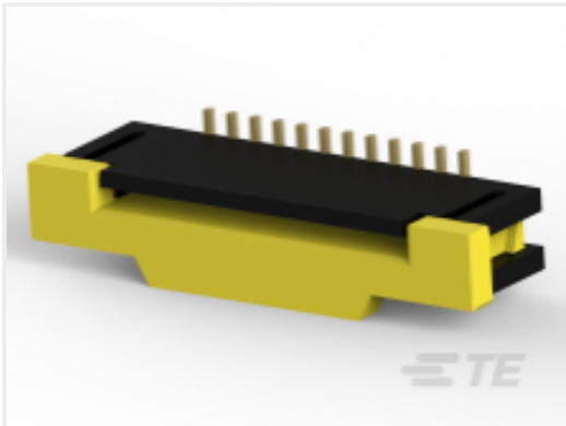
TE Part # 1-1734248-2 1.0 FPC, ZIF V/T, SMT, 12P
