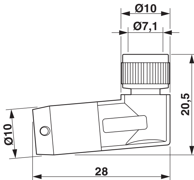
尺寸图
