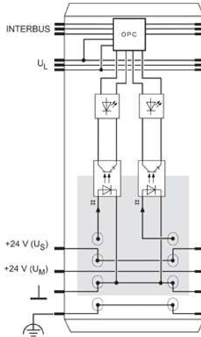
结构框图
