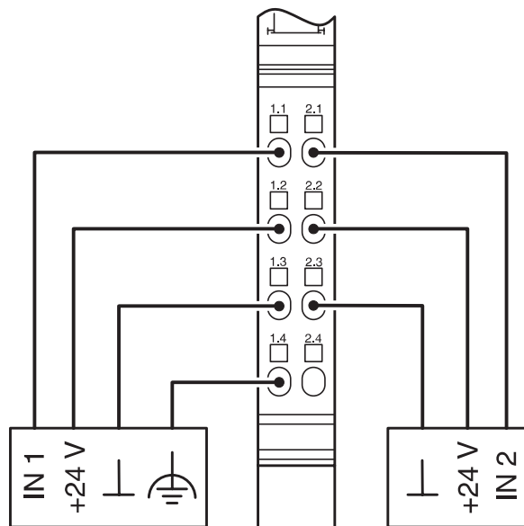
接线图
