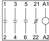
B6(7)-30-01 ... BC6(7)-30-01 ...
