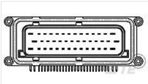
TE Part #1-967280-1 MESSERLEISTE MIX42P
