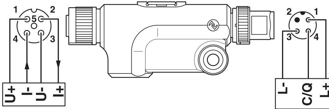
接线图
