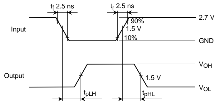
图 2 t_{pLH} , t_{pHL}
