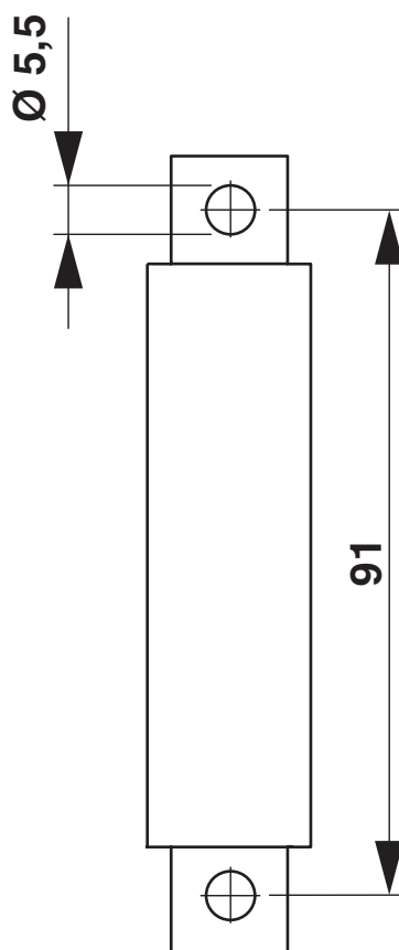
尺寸图
