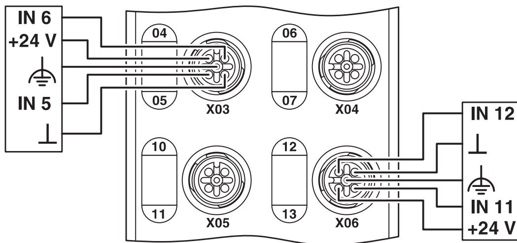
接线图
