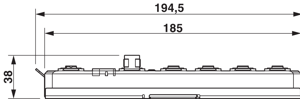
尺寸图
