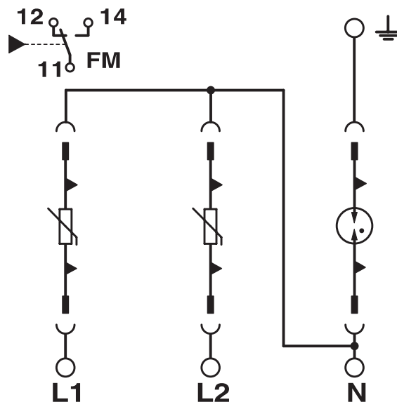
电路图
