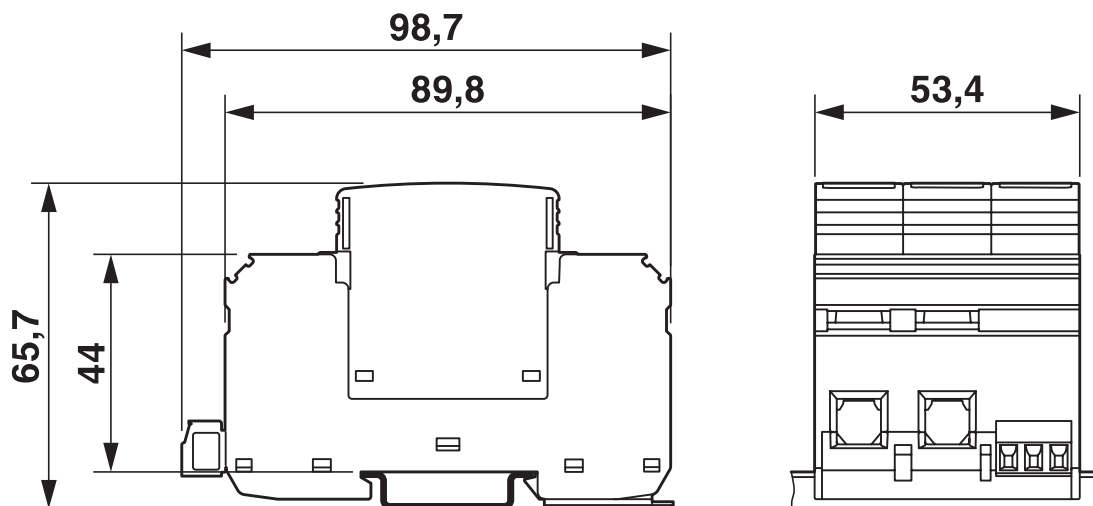
尺寸图
