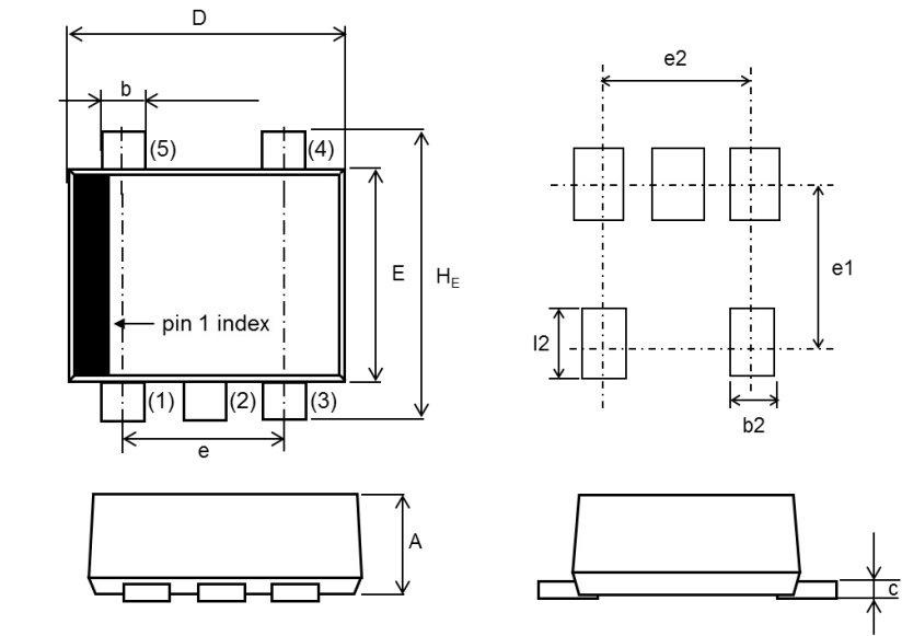
SOT-353T, [SC-113CA], (TUMD5)
