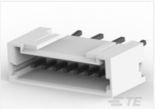
TE Part #2-292207-8 MINI CT SGL DIP V 8P BLACK
