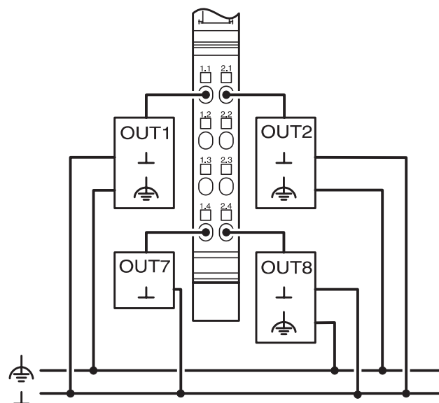
接线图
