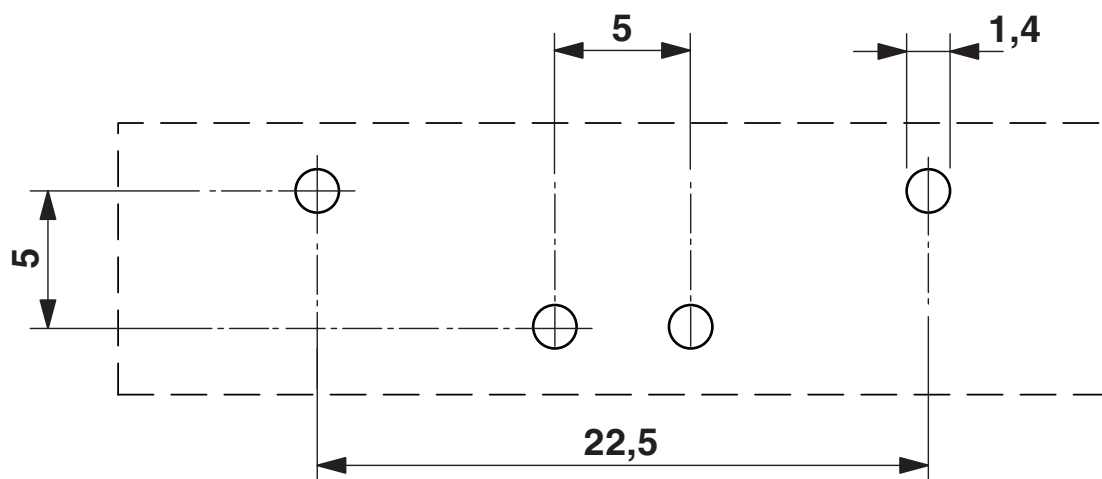
开孔图/焊盘环宽
