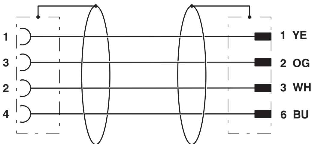
Disposition des contacts du connecteur femelle M12 et du connecteur RJ45
