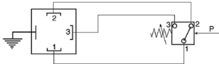
Elektrisches Anschlussbild
