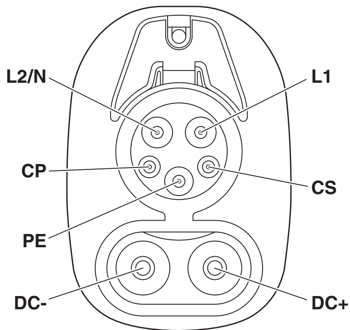
接线图
