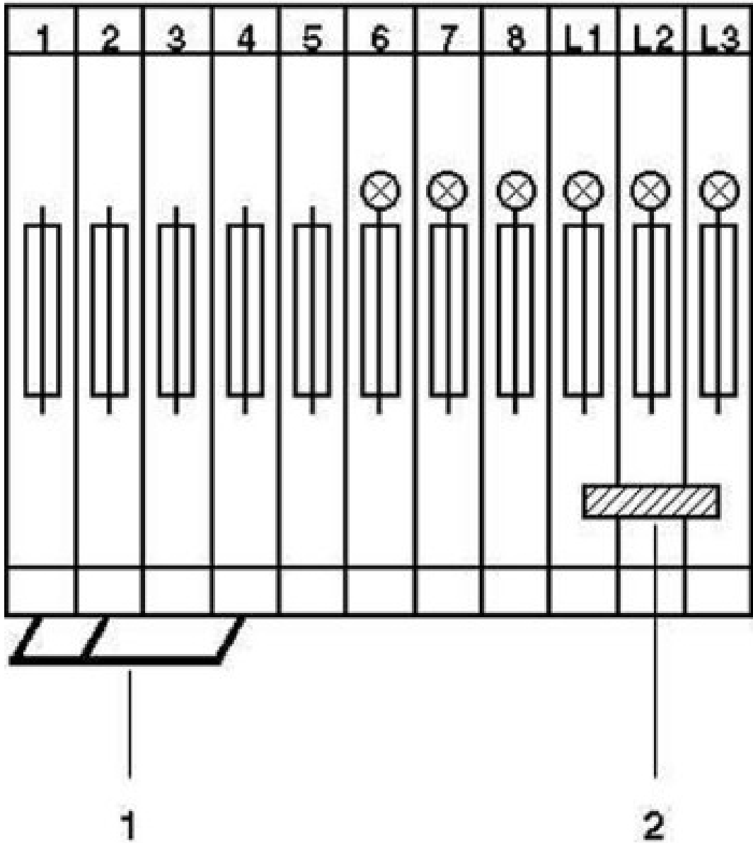
电路图
