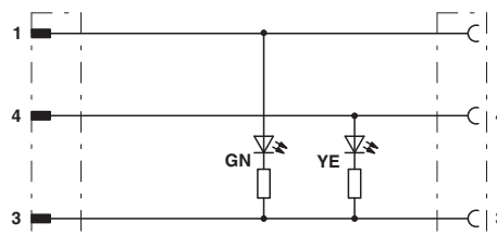
回路図
