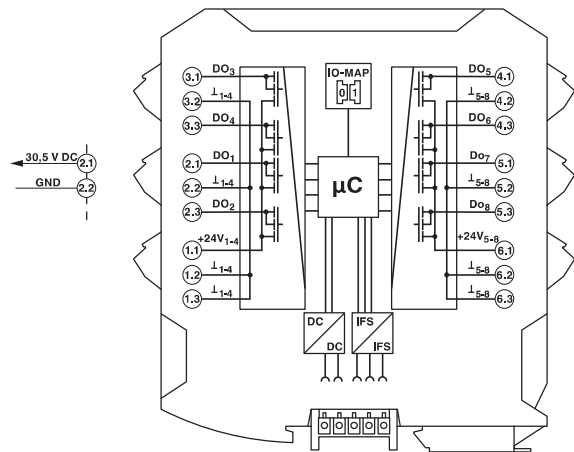
电路图
