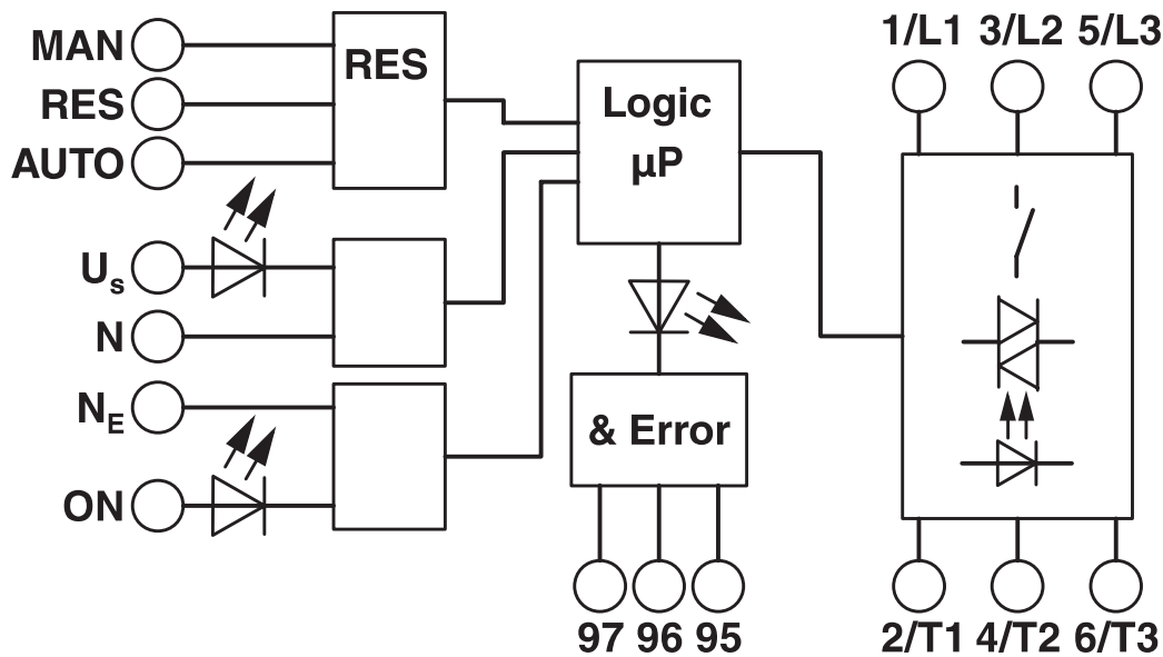
结构框图
