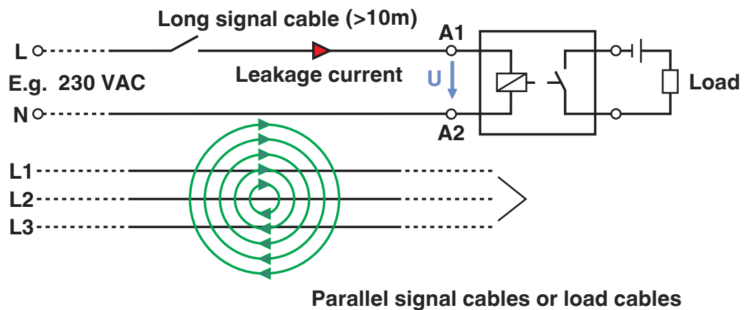
Applikationszeichnung
