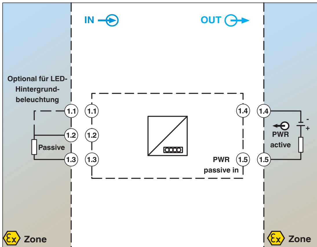
Blockschaltbild FA MCR-EX-DS-I-I-OLP
