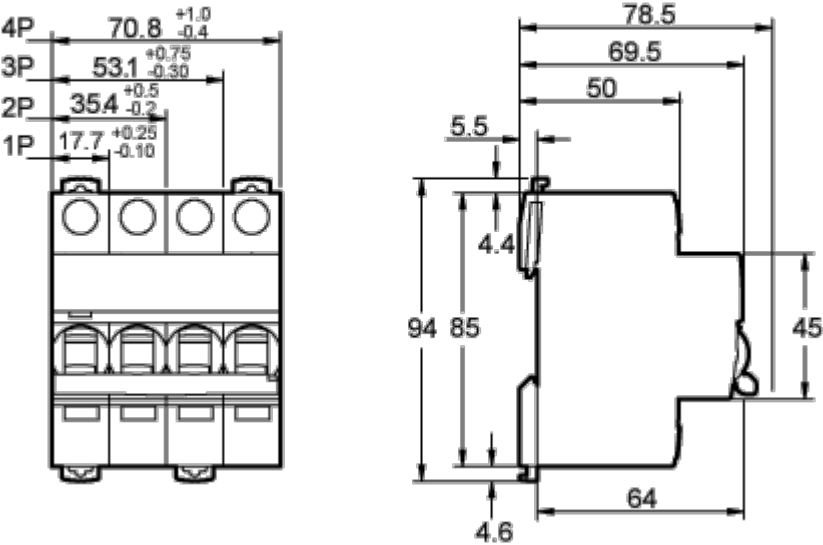
尺寸(mm)
