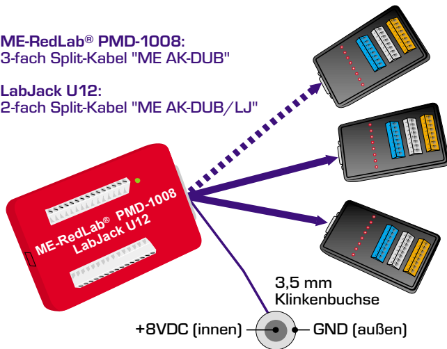
Abb. 2: Anschluß USB-Messboxen
