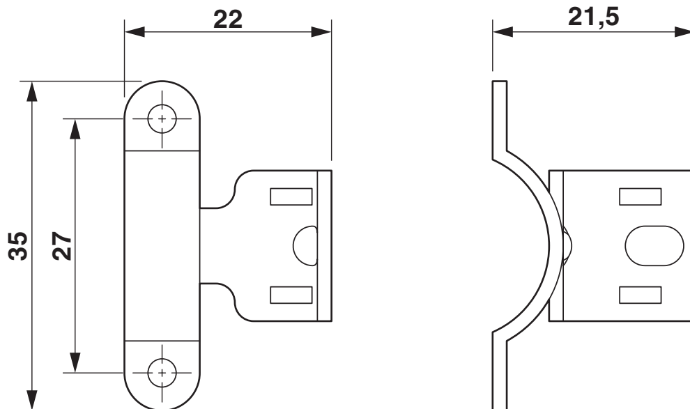
尺寸图
