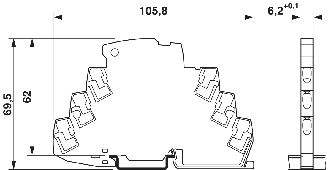
尺寸图
