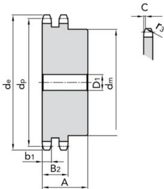
Disegno Tecnico 2D
