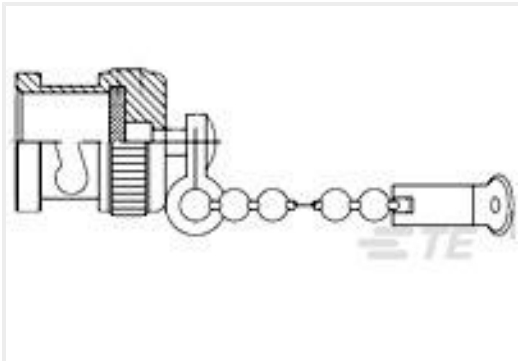
TE Part #1-1337524-0 BNC Plg DCap & Chn Nickel Pltd
