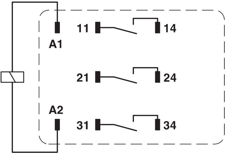
电路图
