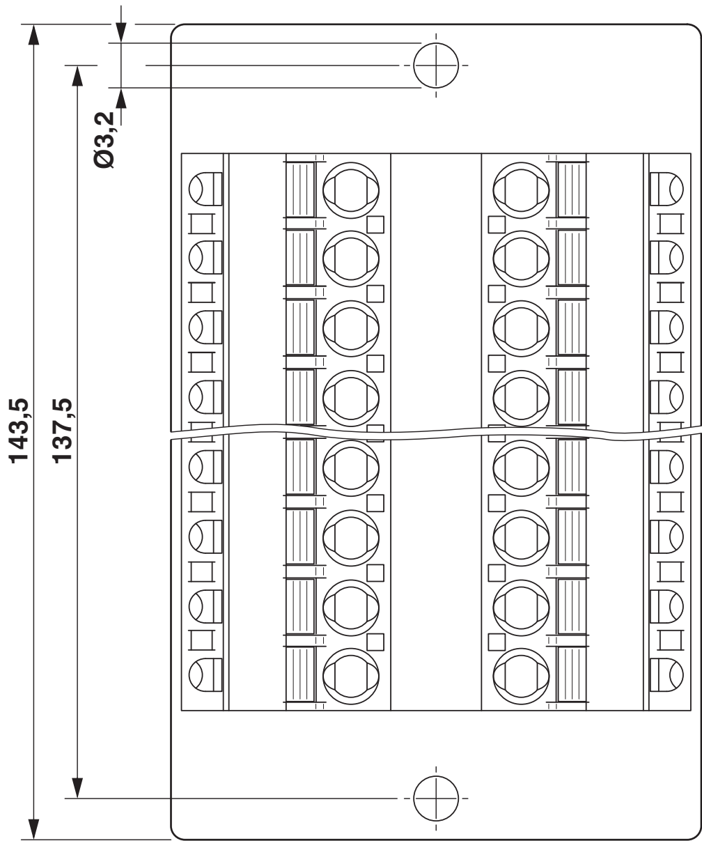
尺寸图
