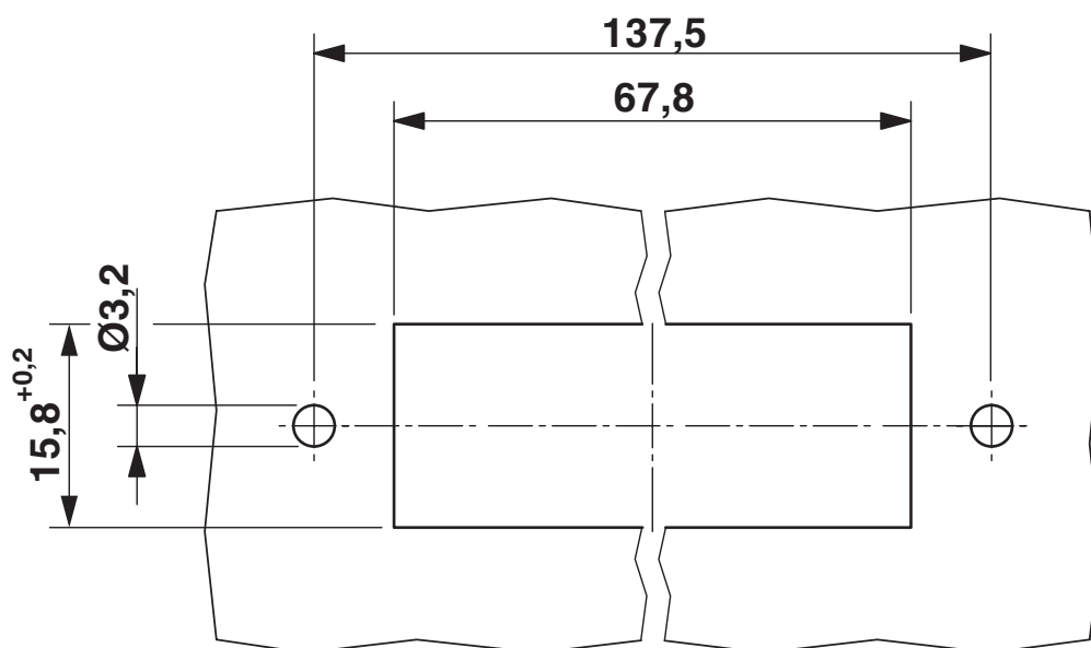
尺寸图
