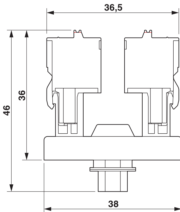
尺寸图
