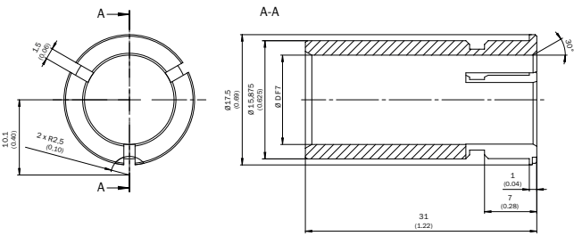
尺寸圖 (尺寸 (mm))
