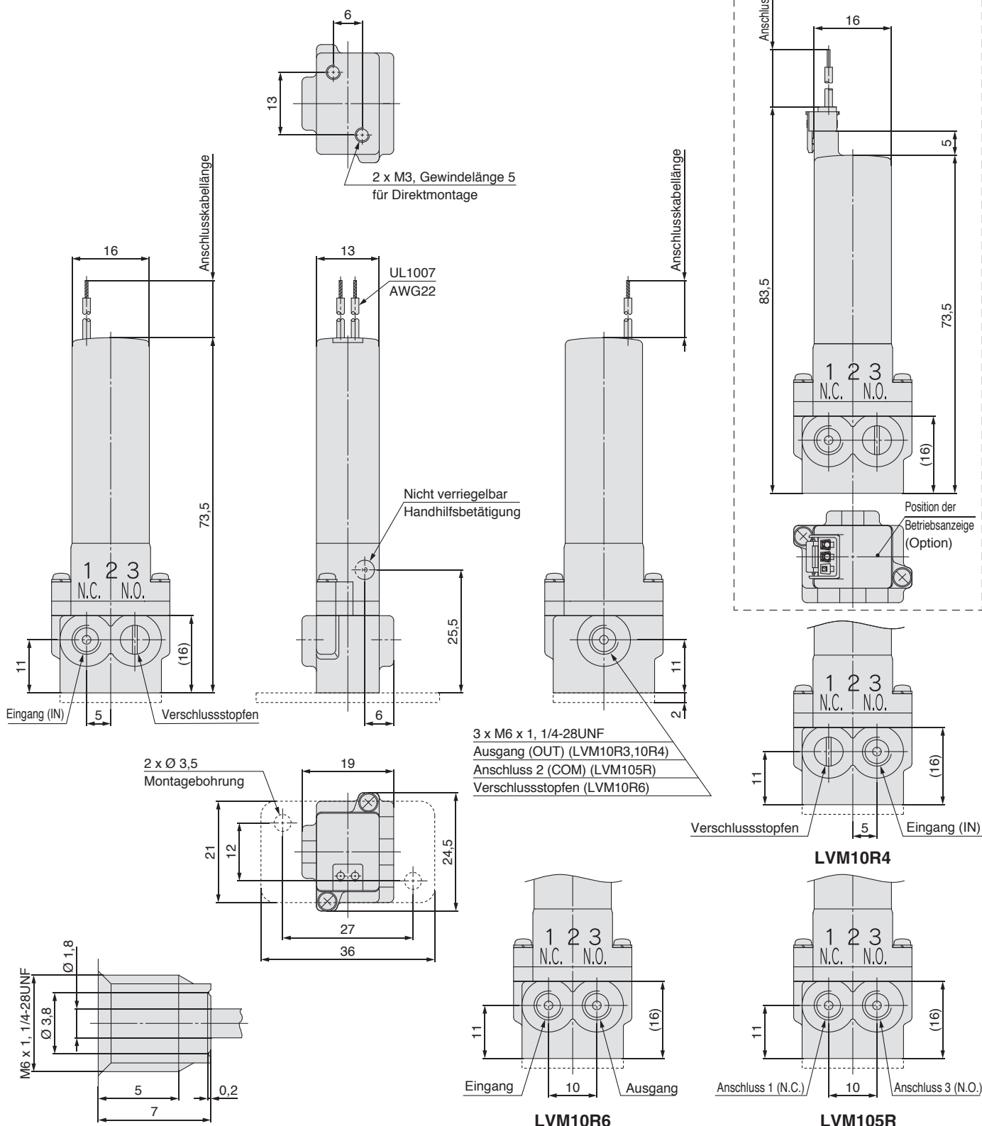
Gewinde-Detail
