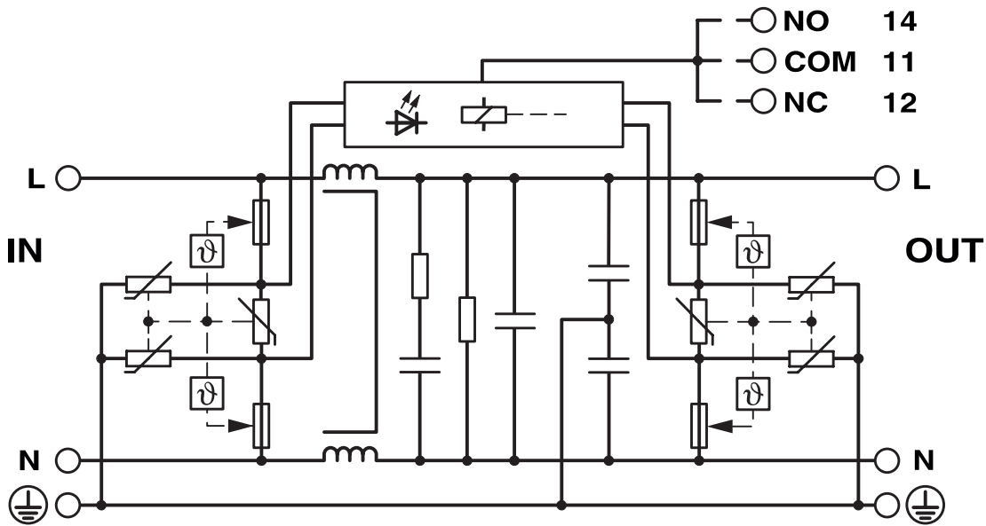
电路图
