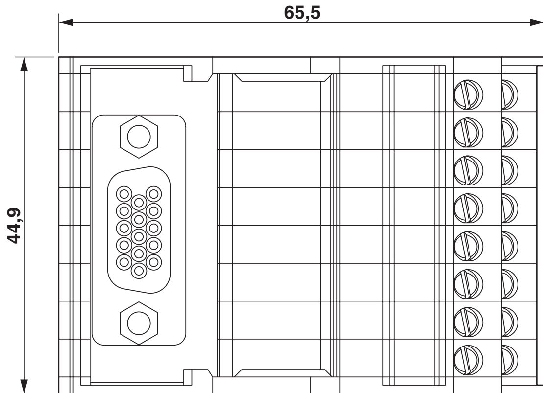
尺寸图
