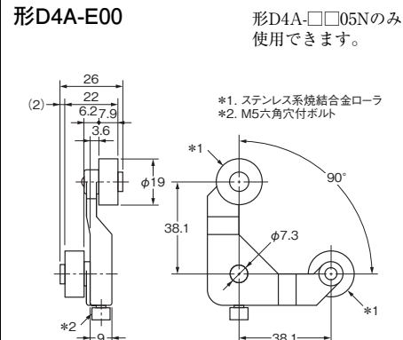
フォーク・レバー・ロック形 形D4A-E00
