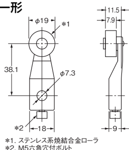
ローラ・レバー形 形D4A-B06
