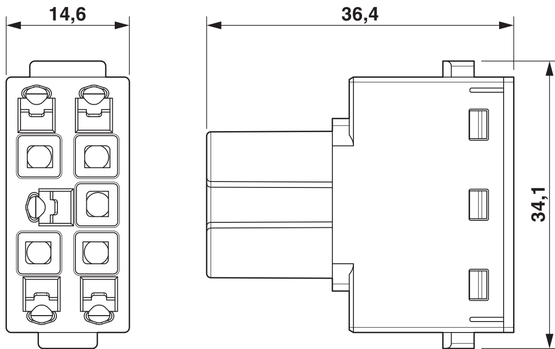
尺寸图
