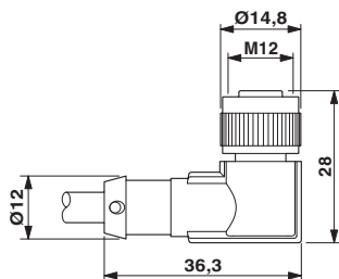
M12ソケットx 1、アングル型
