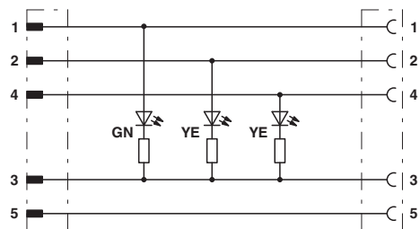
M12コネクタ/ソケットのコンタクトアサイン、LED 3点付き
