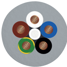
PUR、ハロゲンフリー、極細撚線、耐溶接ス パーク、グレー [802]
