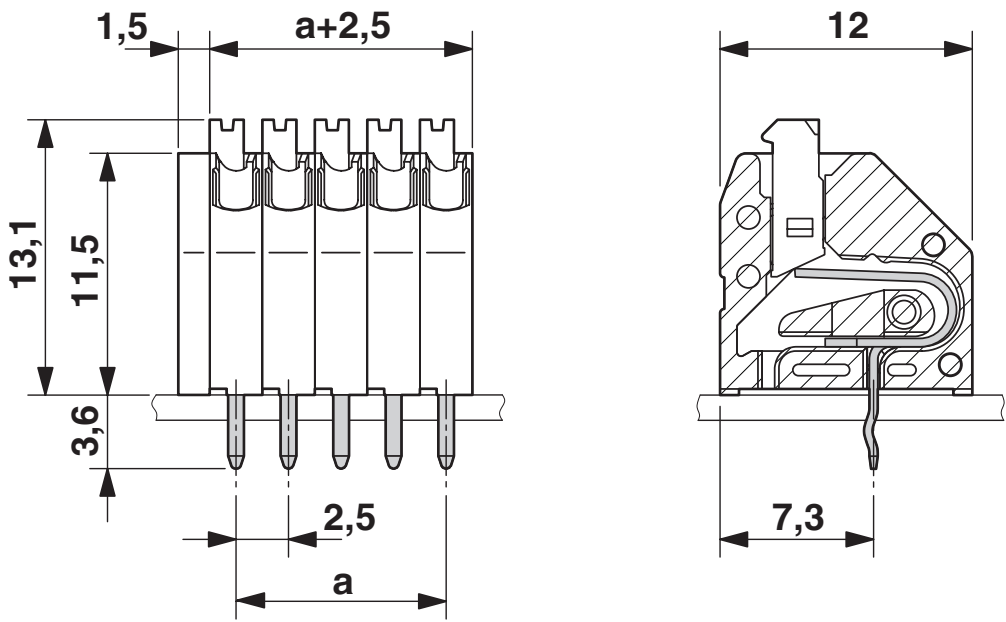
尺寸图
