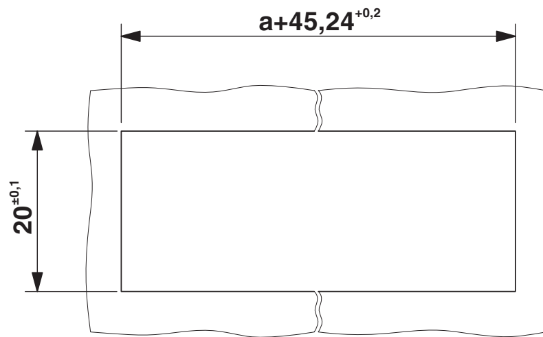
尺寸图
