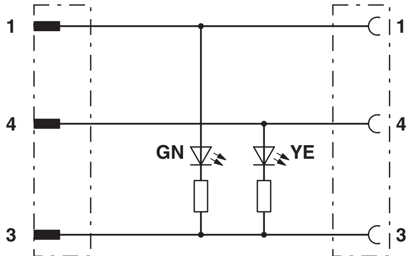
Schaltplan
